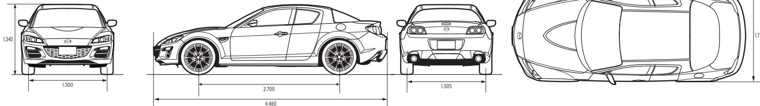
DIMENSIONES (mm)
